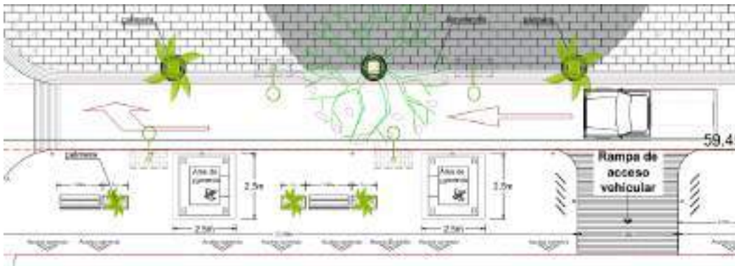
Figura 12. Diseño de calle Cerrada Miguel Hidalgo, Centro de Ixtapaluca.
